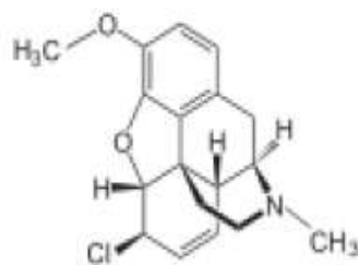
\alpha -Chlorocodide
