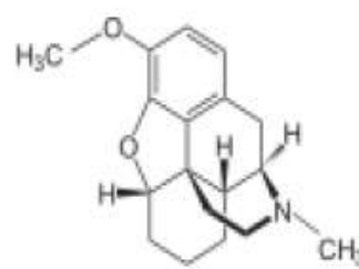
Desocodeine
