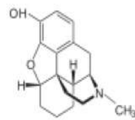
Desomorphine
